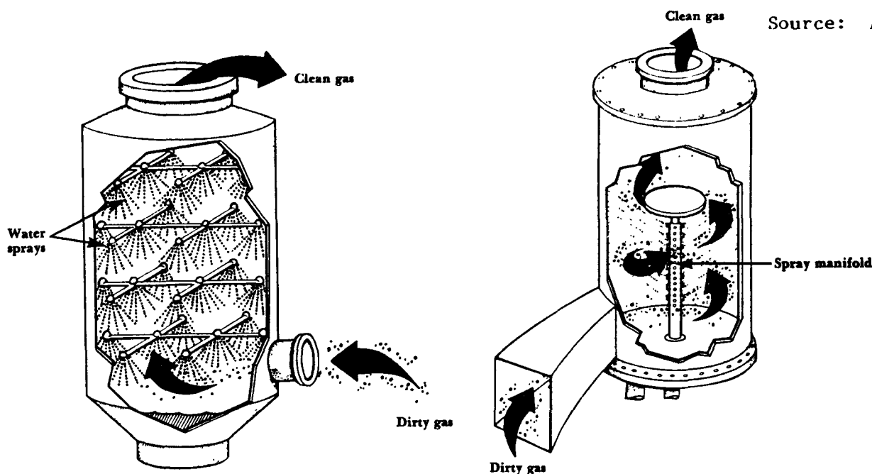
a. Simple Spray Tower
