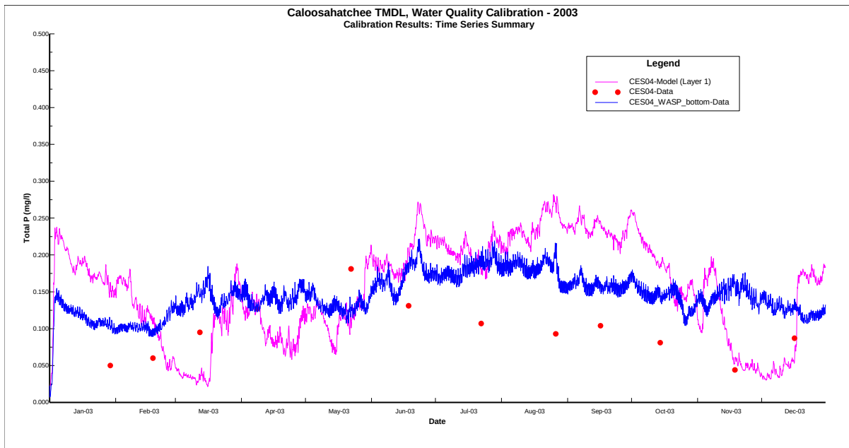
068_Tot P_CES04_Bottom
