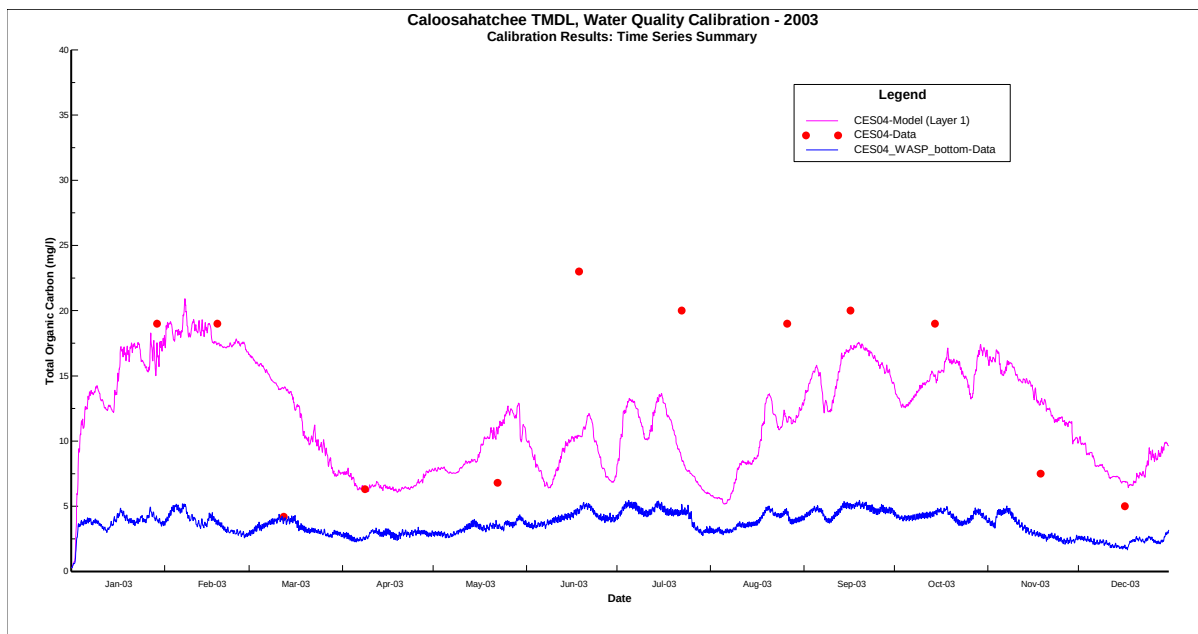
108_TOC_CES04_Bottom
