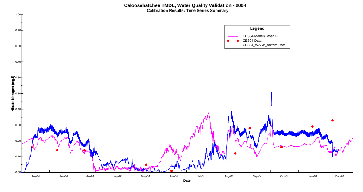
100_NO3-N_CES04__Bottom
