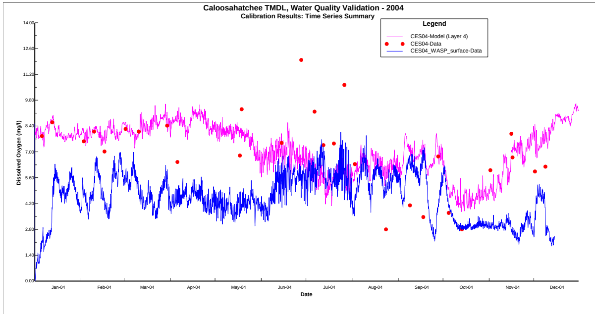
050_DO_CES04_Surface
