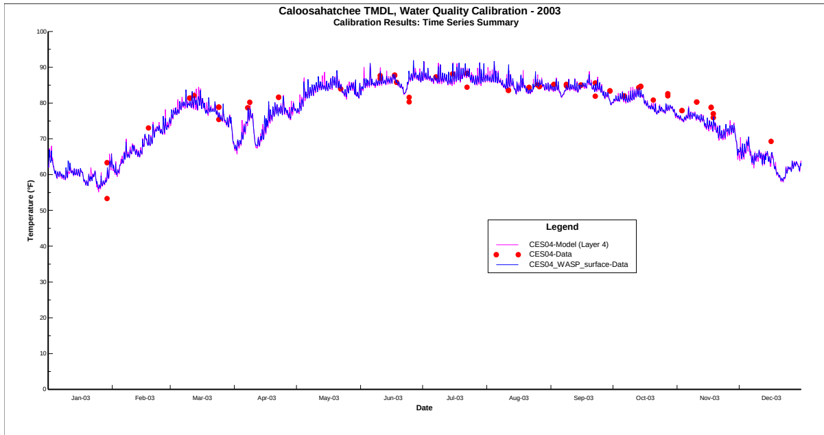
Temp_CES04_Surface
