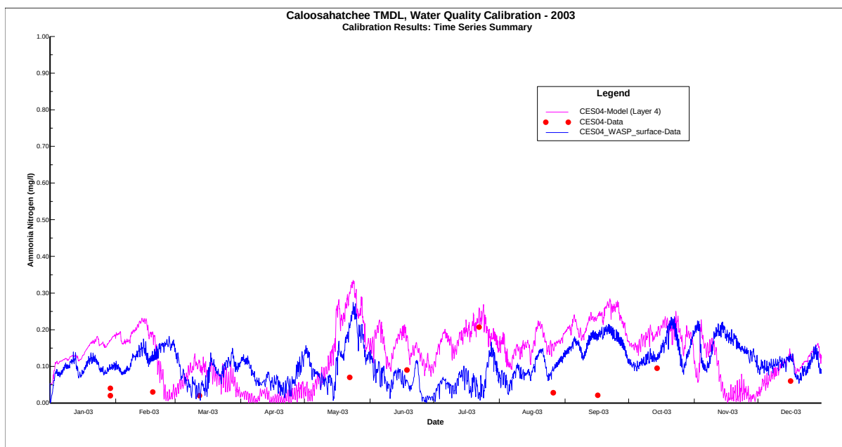
091_NH4-N_CES04_Surface
