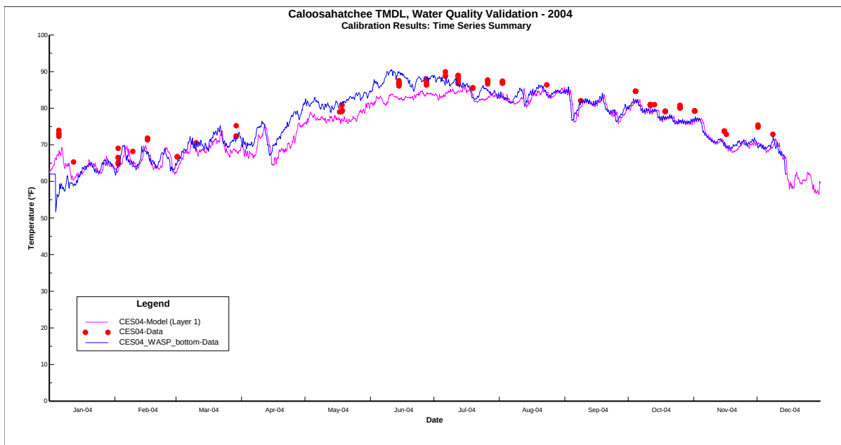
029_Temp_CES04__Bottom
