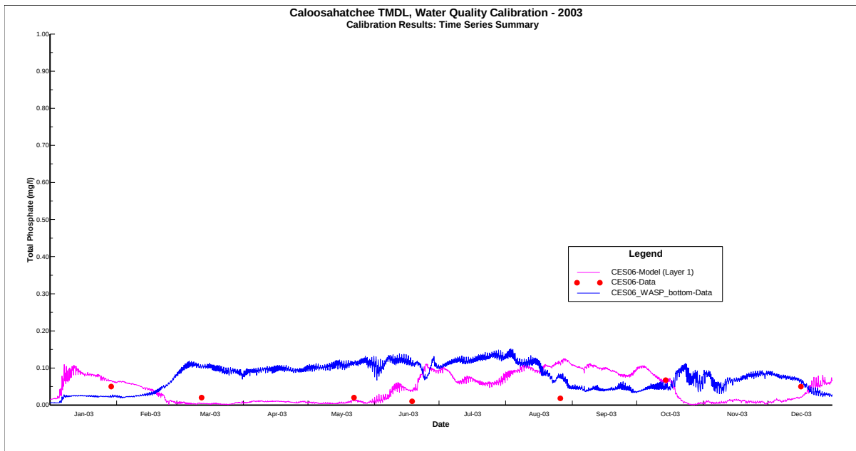
078_TPO4-P_CES06_Bottom
