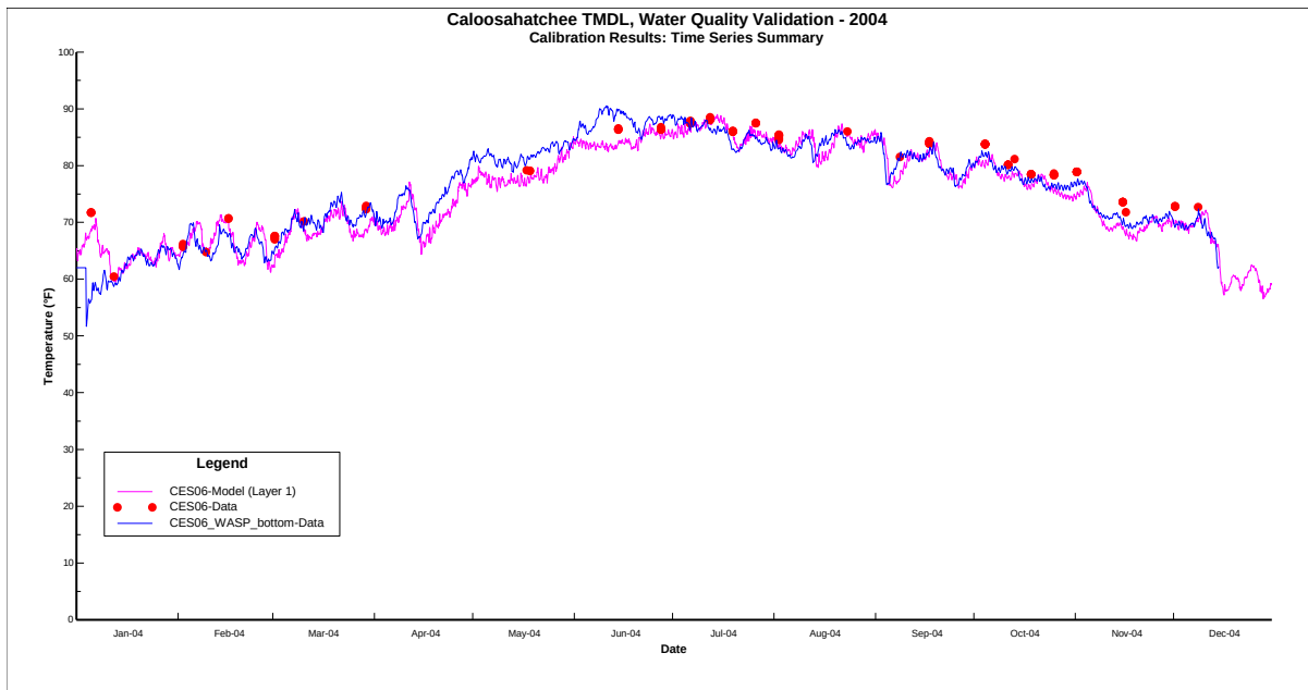
033_Temp_CES06__Bottom
