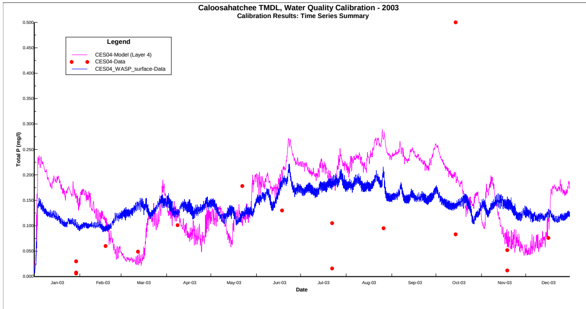
067_Tot P_CES04_Surface
