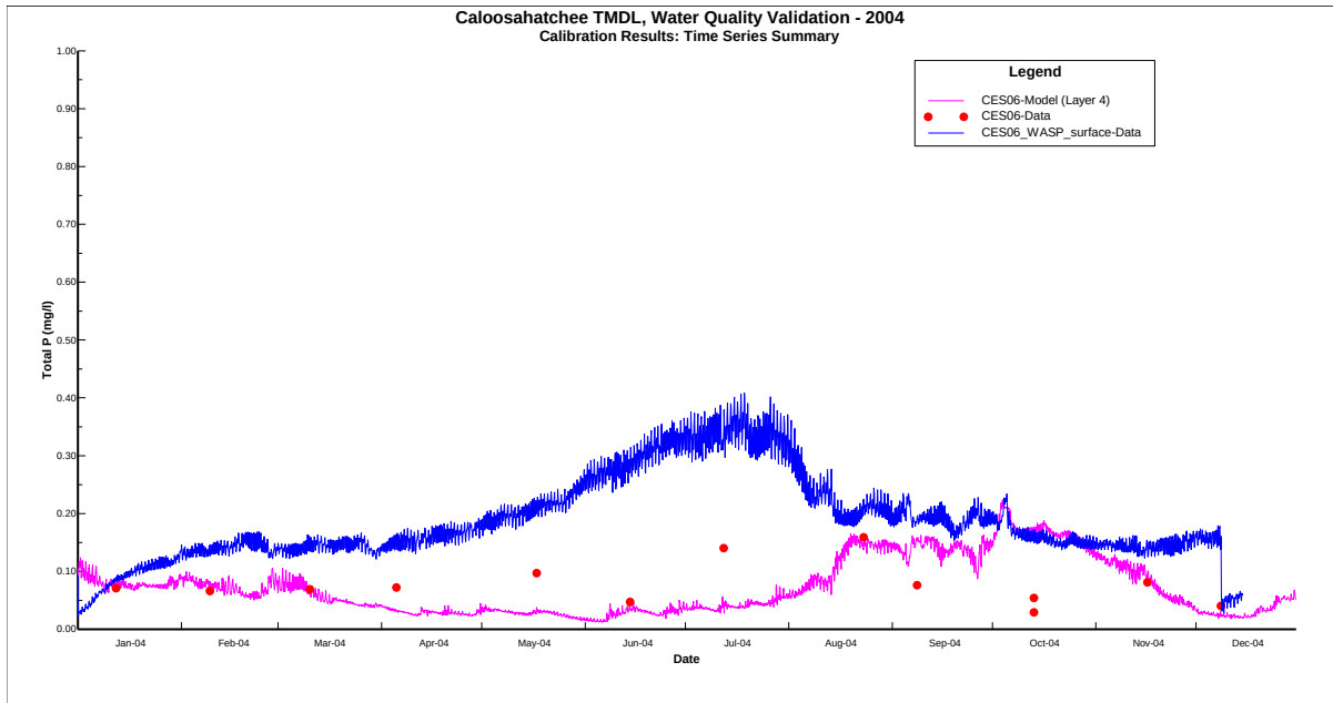
069_Tot P_CES06__Surface
