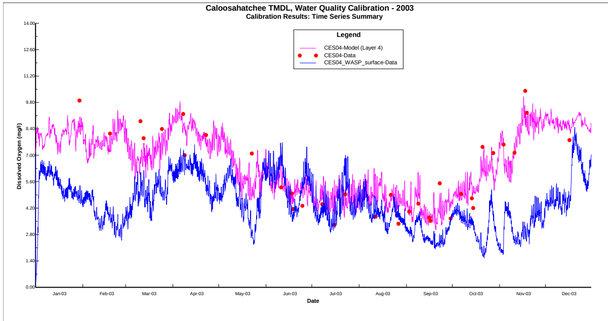
DO_CES04_Surface
