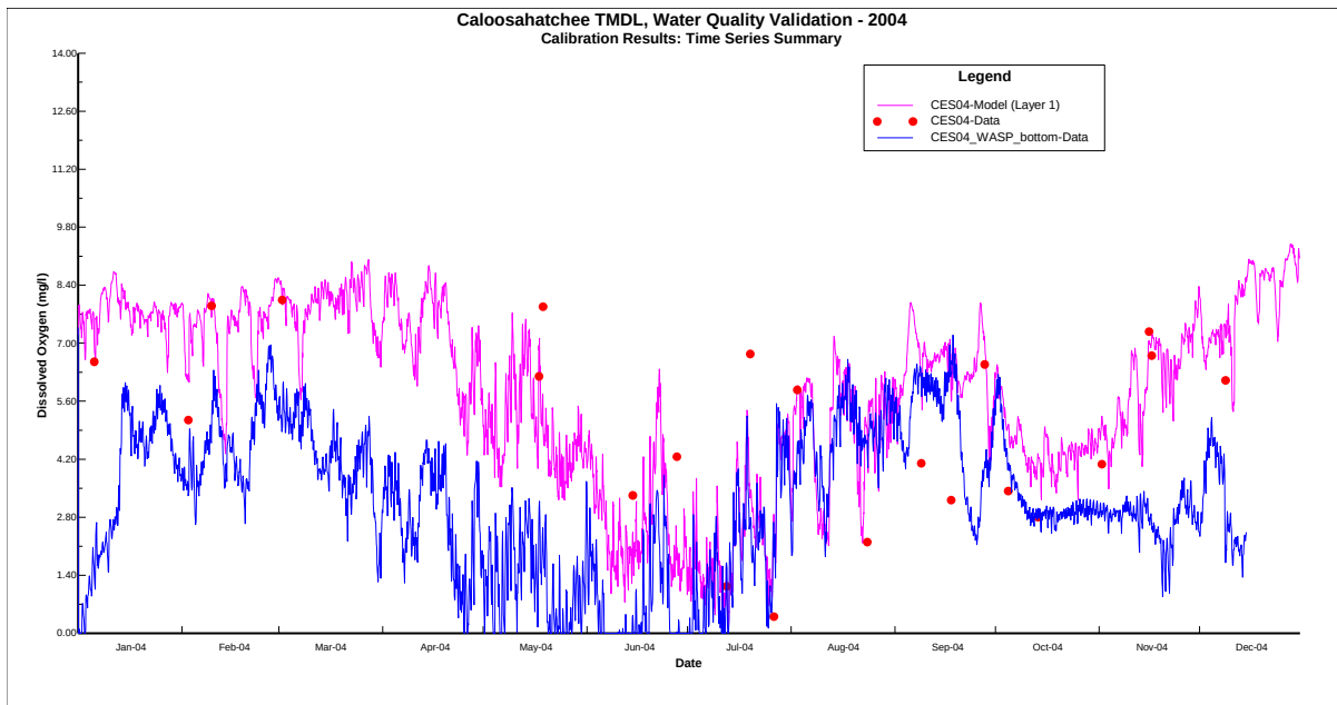
051_DO_CES04_Bottom
