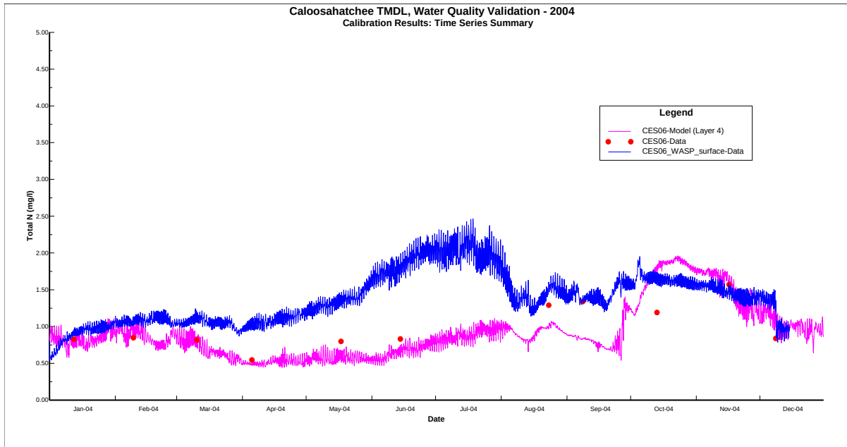
085_Tot N_CES06__Surface
