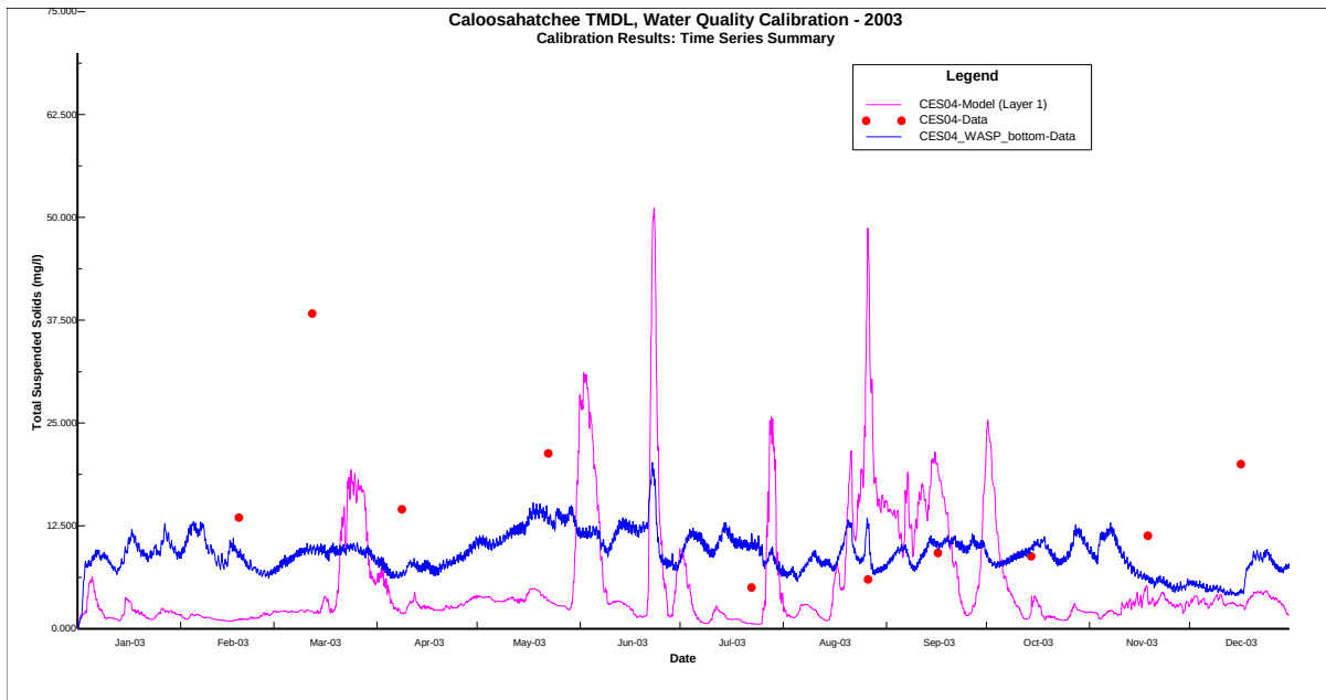
116_TSS_CES04_Bottom
