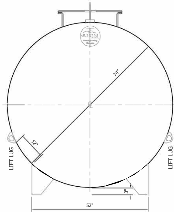
END ELEVATION
