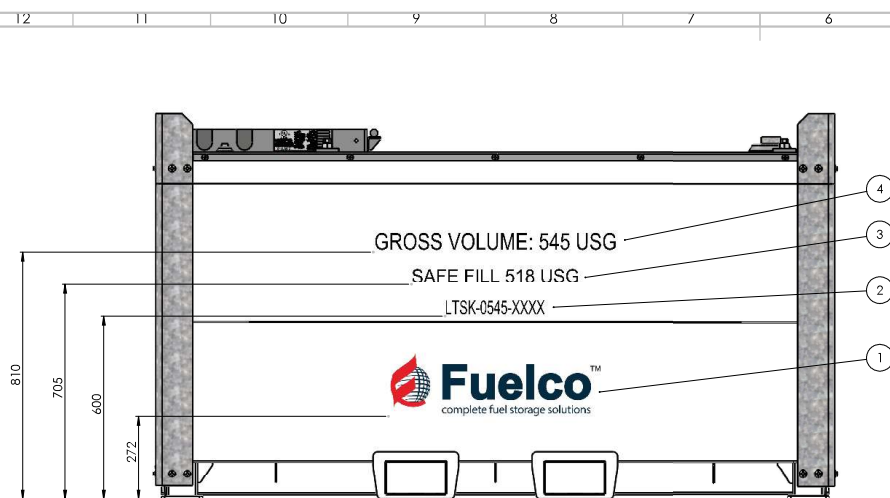
LTSK-0545 - LHS & RHS - DECAL MAP
