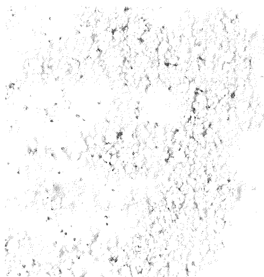
Forams
