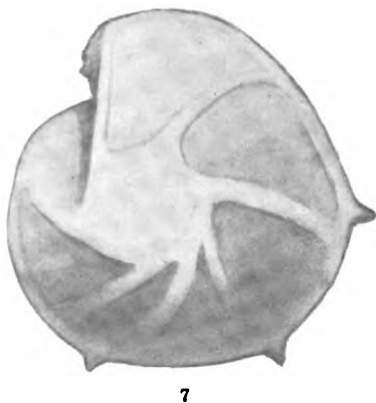
MIOCENE FORAMINIFERA.
