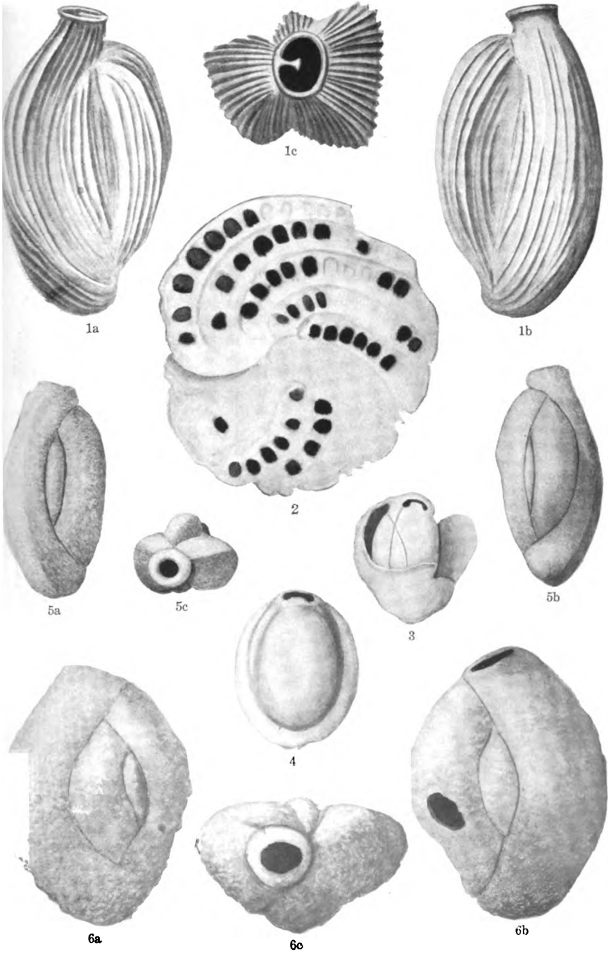
PLIOCENE FORAMINIFERA.
