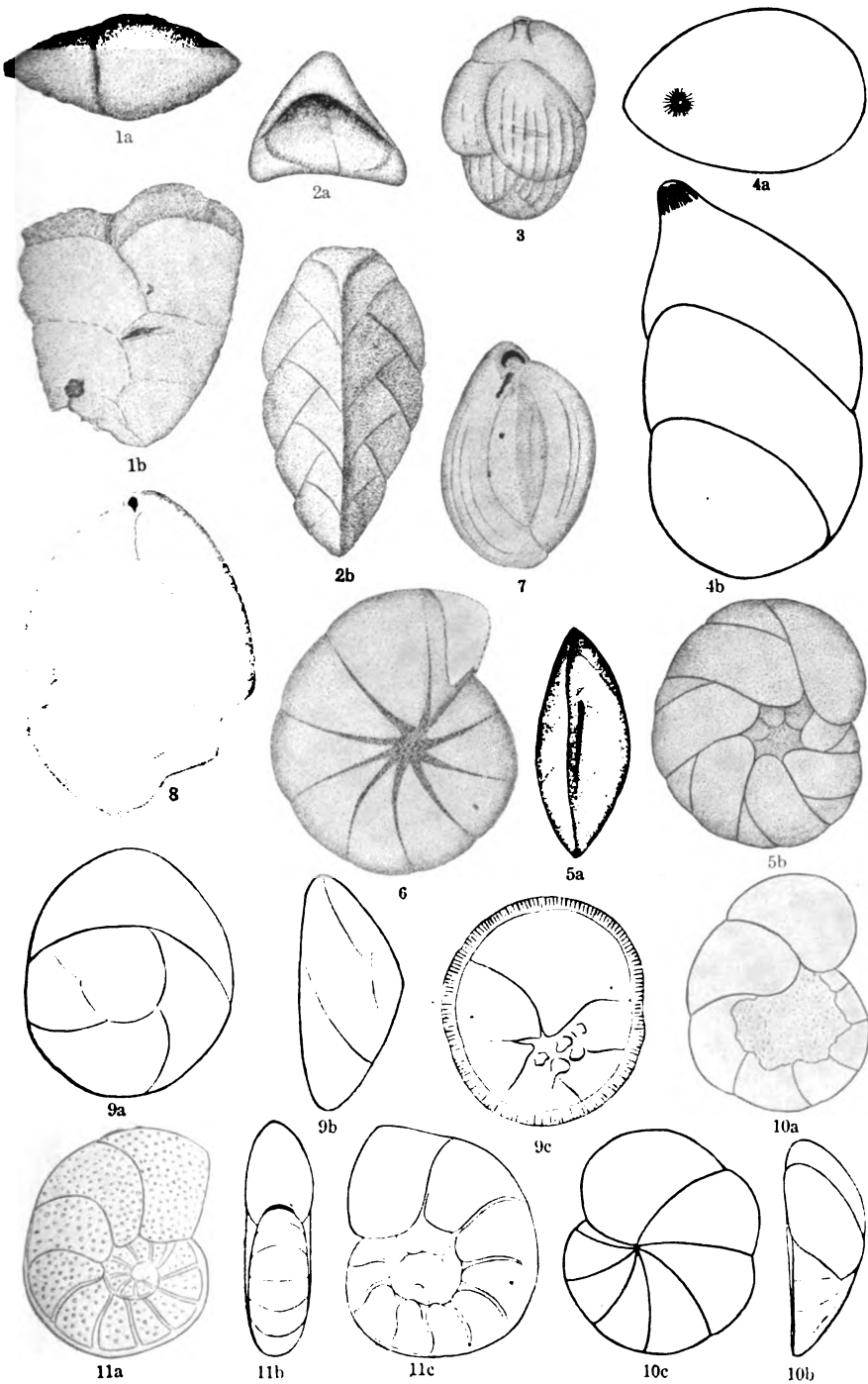
PLIOCENE FORAMINIFERA.
