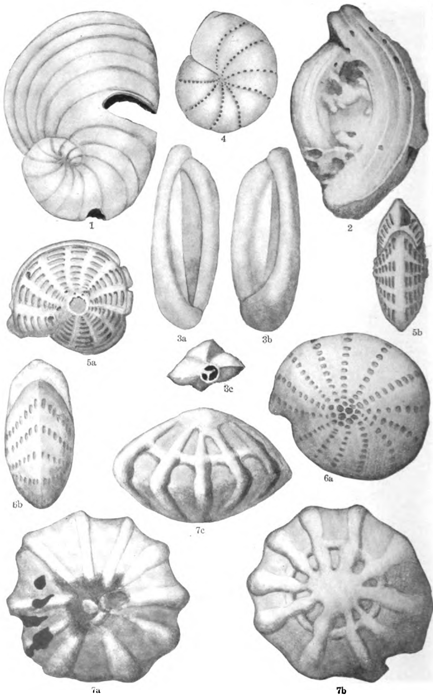
PLIOCENE FORAMINIFERA
