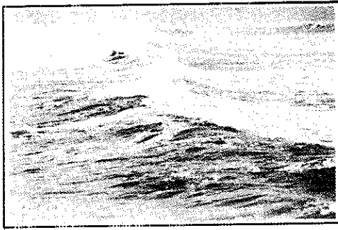
SPILLING BREAKER
