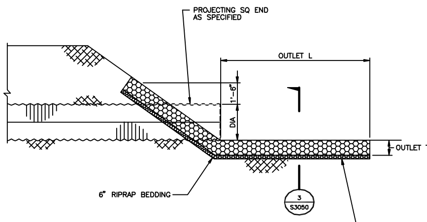
OUTLET END SEE RIPRAP TABLE
