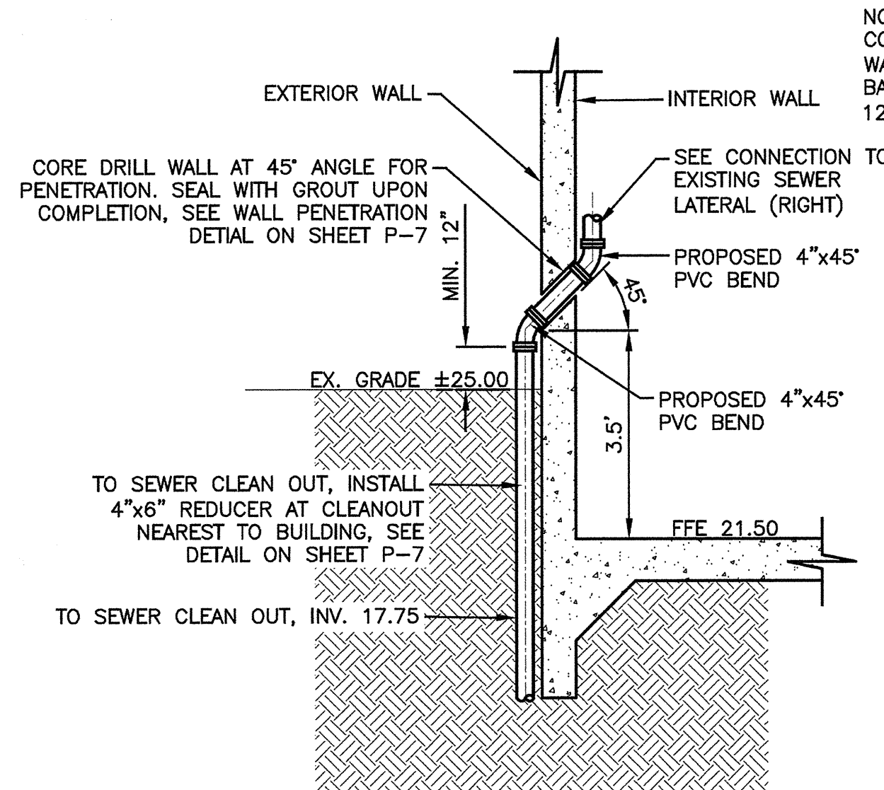
SIDE VIEW SEWER LATERAL WALL PENETRATION SCALE: N.T.S.
