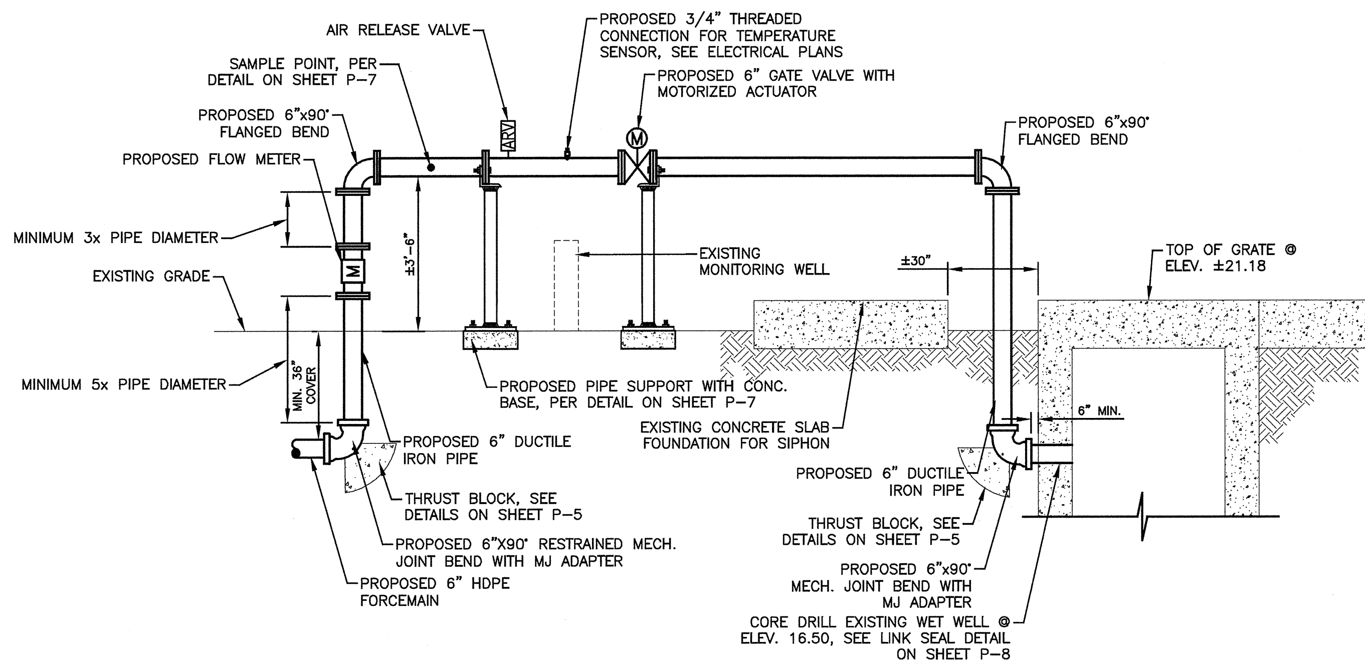
SECTION SCALE: 3/8"=1'-0"
